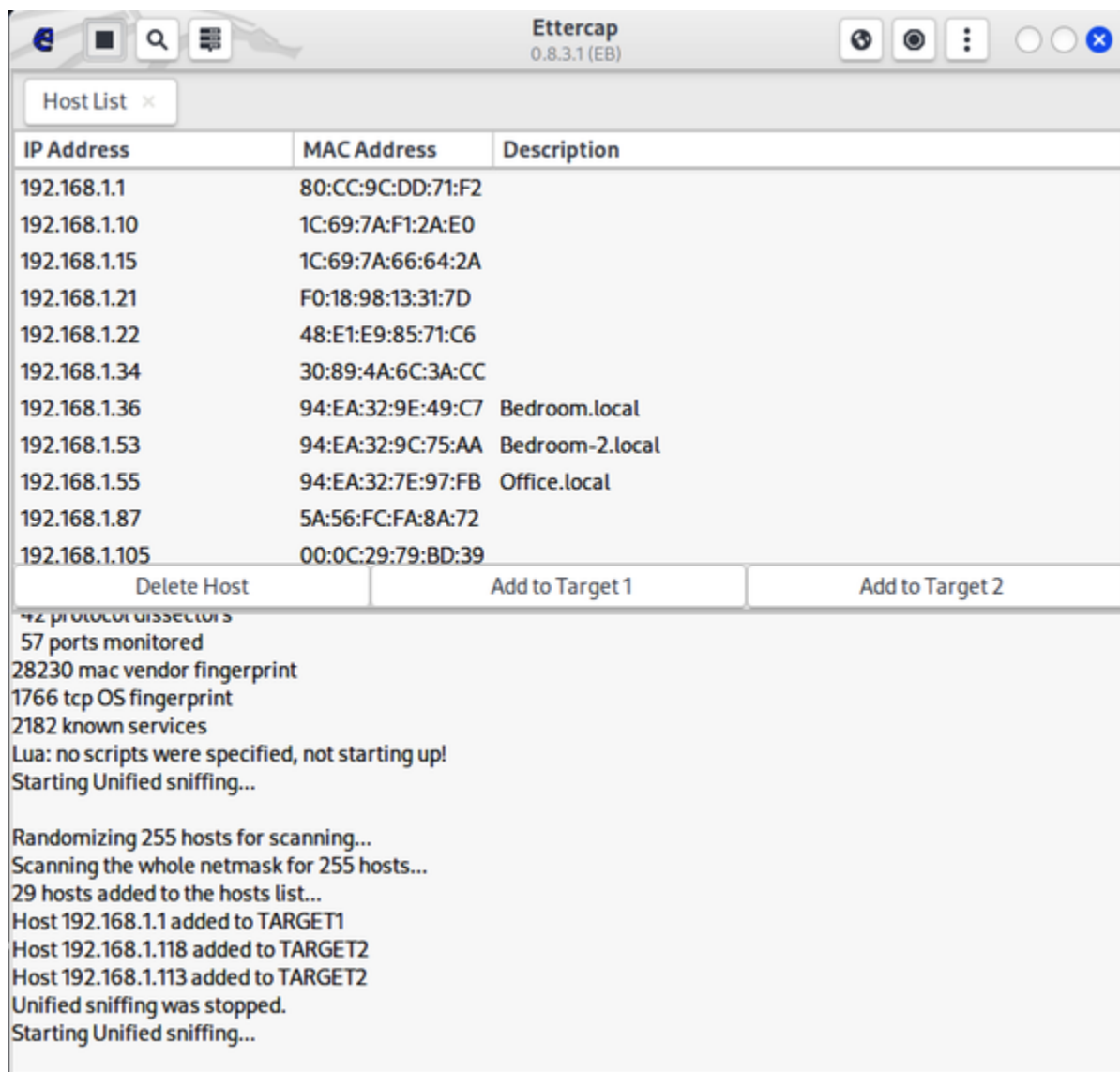
Figure 2-8. Using Ettercap
