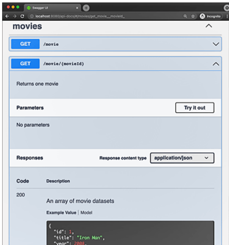
Figure 10.10 Swagger UI
