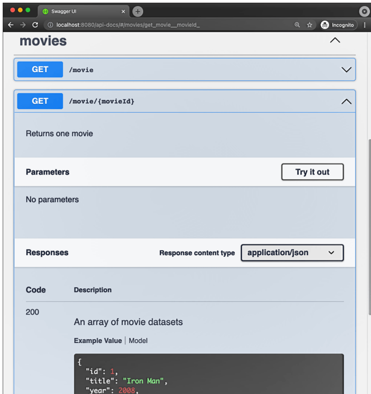
Figure 10.10 Swagger UI
